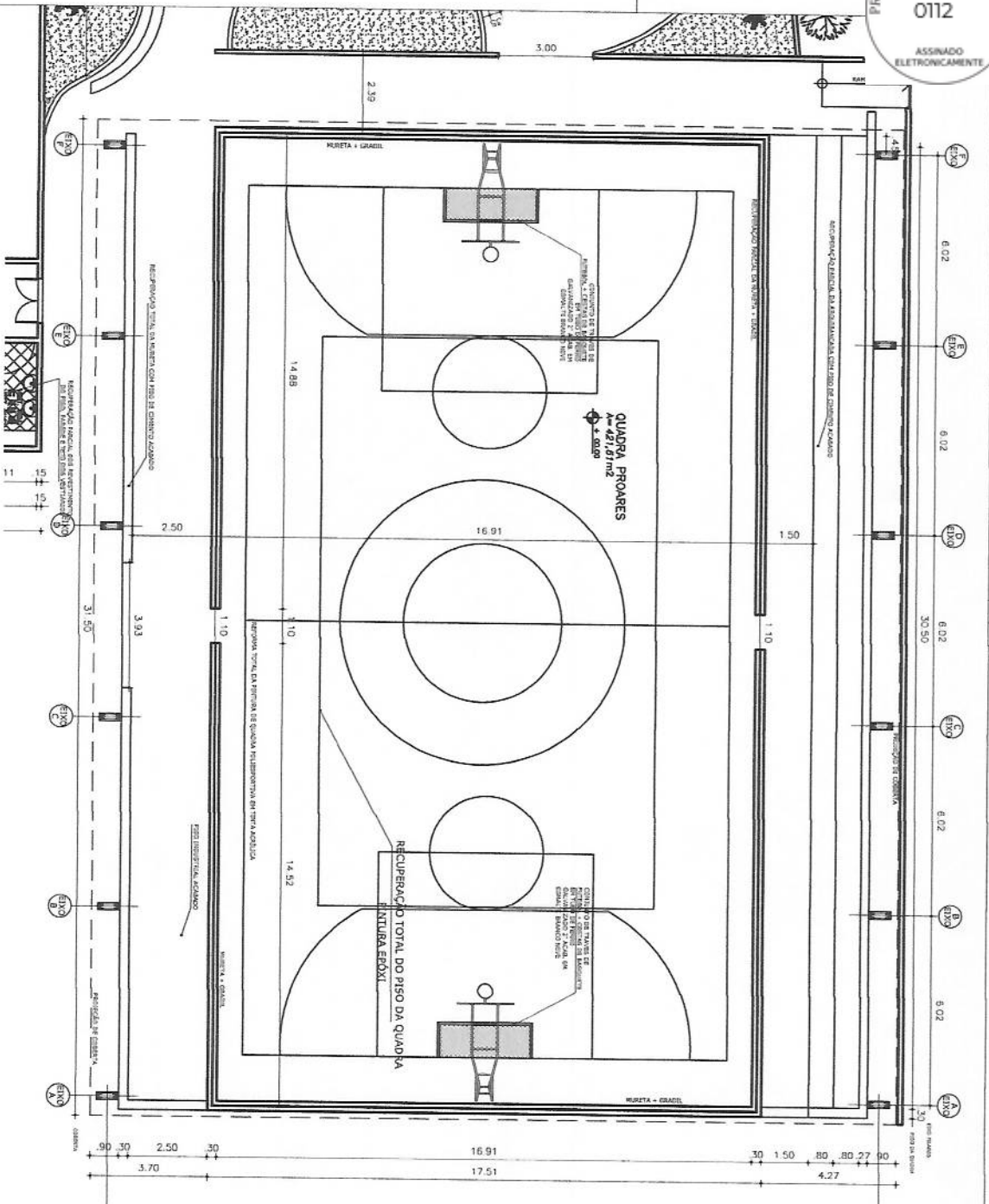
01 PLANTA BAIXA - QUADRA POLIESPORTIVA esc.: 1:100
