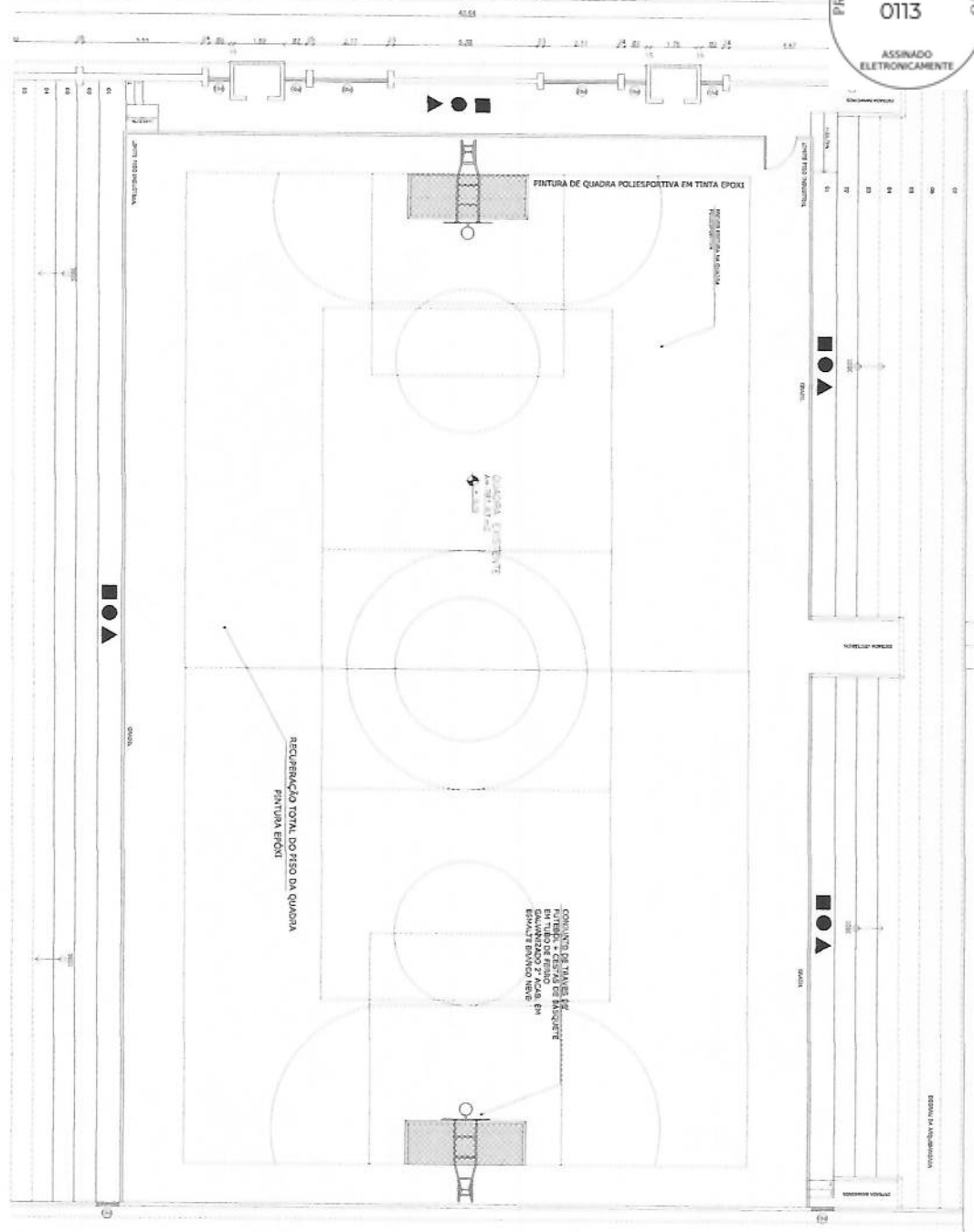
01 PLANTA BAIXA - QUADRA POLIESPORTIVA 1/50
